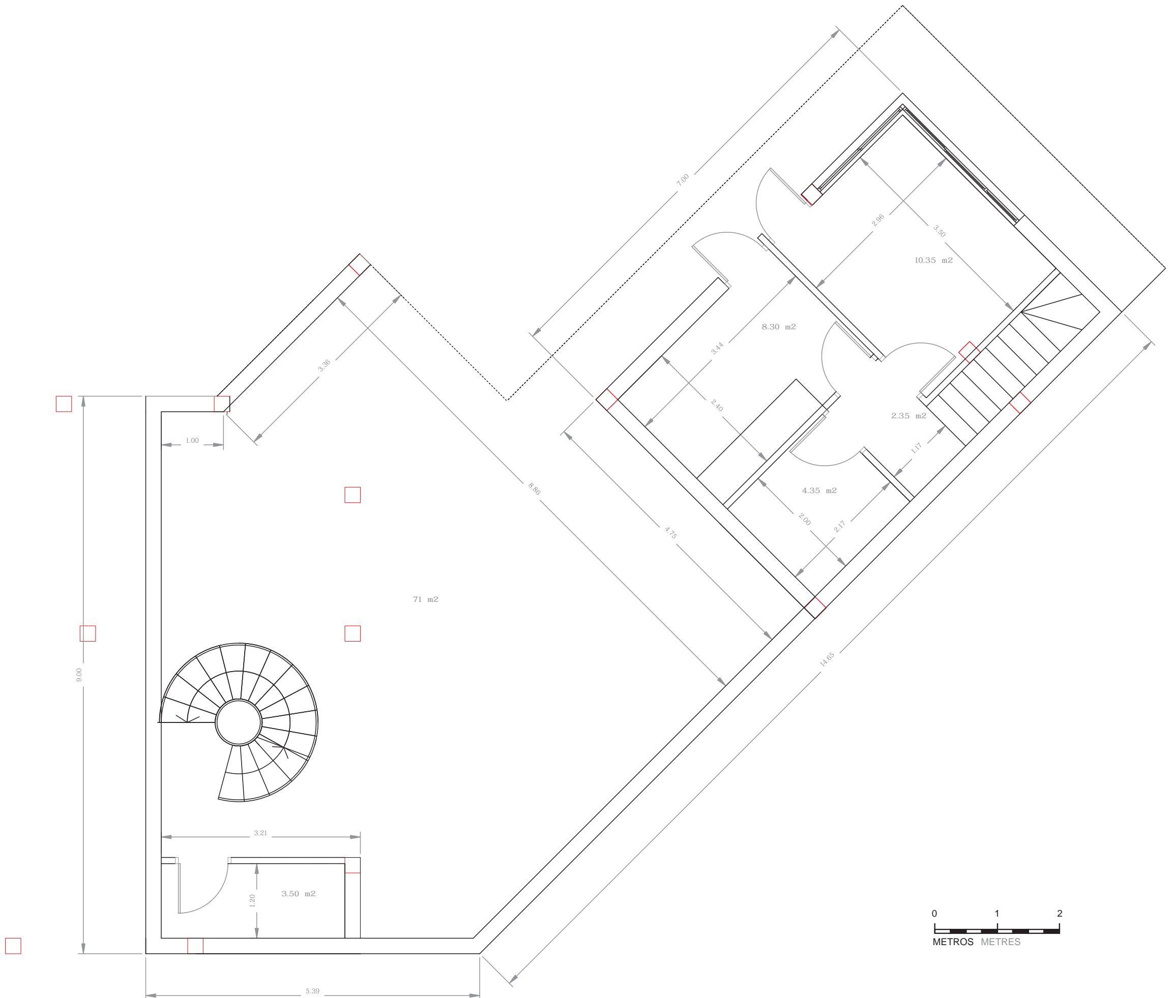
PLANTA NIVEL SEMISÓTANO LEVEL SEMI-BASEMENT
